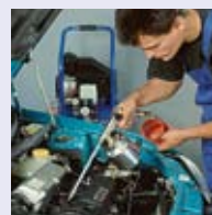
Sprühpistole 120-500 l/min, 6-10 bar
